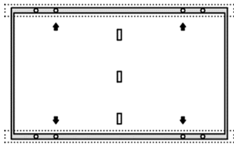
Figure 3 : Montage avec fixation sur le côté long avec les 4 trous intérieurs pour le montage des boulons. Profilé en acier parallèle au côté long. Charge maximale : Avant \leq 2400 Pa ; Arrière \leq 1600 Pa
