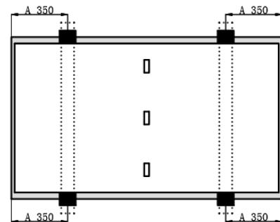
Figure : 7 : Montage avec 4 étriers sur le long coté. Profilé en acier perpendiculaire au côté long. Etrier : Largeur = 40-50mm, Hauteur = 30mm. Distance A = 350 \pm 30 mm. Charge maximale : Avant \leq 3600 Pa, Arrière \leq 1600 Pa
