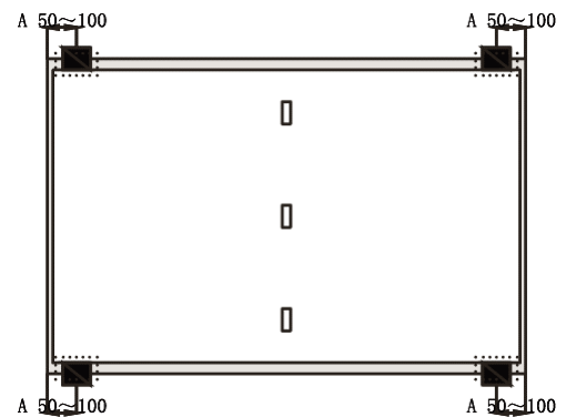
Figure : 8 : Montage avec 4 étriers sur le long coté. Profilé en acier dans les angles. Etrier : Largeur = 40-50mm, Hauteur = 30mm. Distance A = 50-100mm. Charge maximale : Avant \leq 1600 Pa, Arrière \leq 1600 Pa
