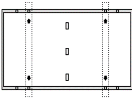
Figure 4 : Montage avec fixation sur le côté long avec les 4 trous intérieurs pour le montage des boulons. Profilé en acier perpendiculaire au côté long. Charge maximale : Avant \leq 3600 Pa ; Arrière \leq 1600 Pa
