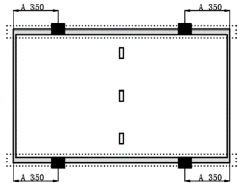
Figure : 6 : Montage avec 4 étriers sur le long coté. Profilé en acier parallèle au côté long. Etrier : Largeur = 40-50mm, Hauteur = 30mm. Distance A = 350 \pm 30 mm. Charge maximale : Avant \leq 2400 Pa, Arrière \leq 1600 Pa
