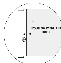
Figure 5 : Vue détaillée d'un trou de mise à la terre
