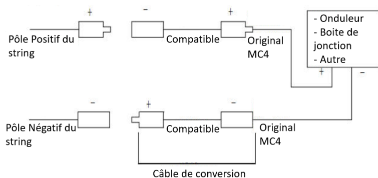
Figure 4 : Câble de conversion
