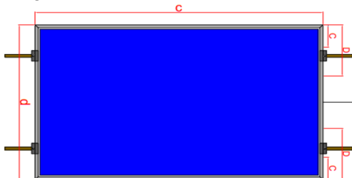
Figure 7 : Limite de pose des étriers sur le côté court du module
