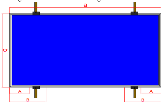
Figure 6 : Limite de pose des étriers sur le côté long du module
