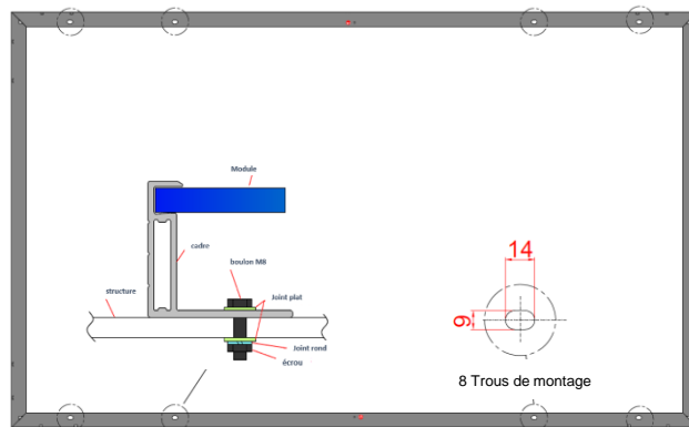
Figure 8 : Montage des panneaux avec vis de fixation
