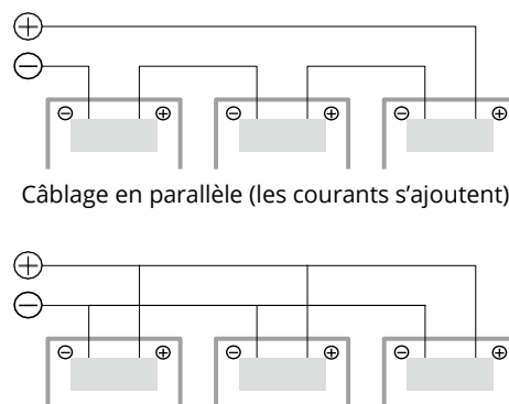
Figure 2 : Schémas électriques des câblages en série et en parallèle
