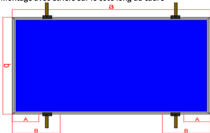
Figure 5 : Limite de pose des étriers sur le côté long du module
