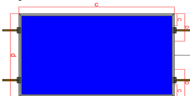
Figure 6 : Limite de pose des étriers sur le côté court du module
