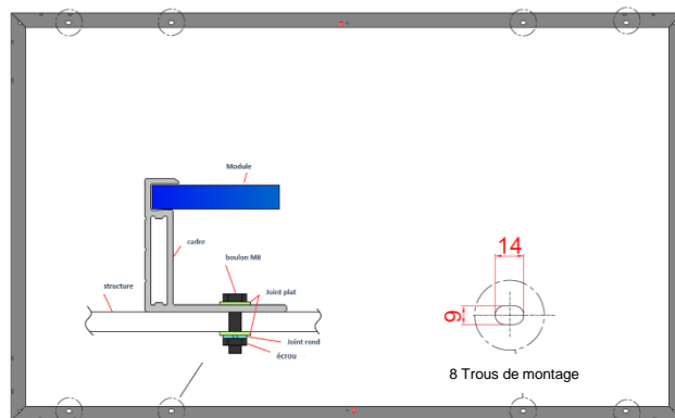
Figure 7 : Montage des panneaux avec vis de fixation
