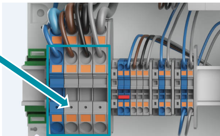
Bornier réseau
